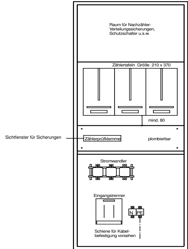
Abb. 4: Niederspannungsverteiler mit Messwandleranlage und Hausanschlussteil (Verdrahtung nach Abb. 3)
