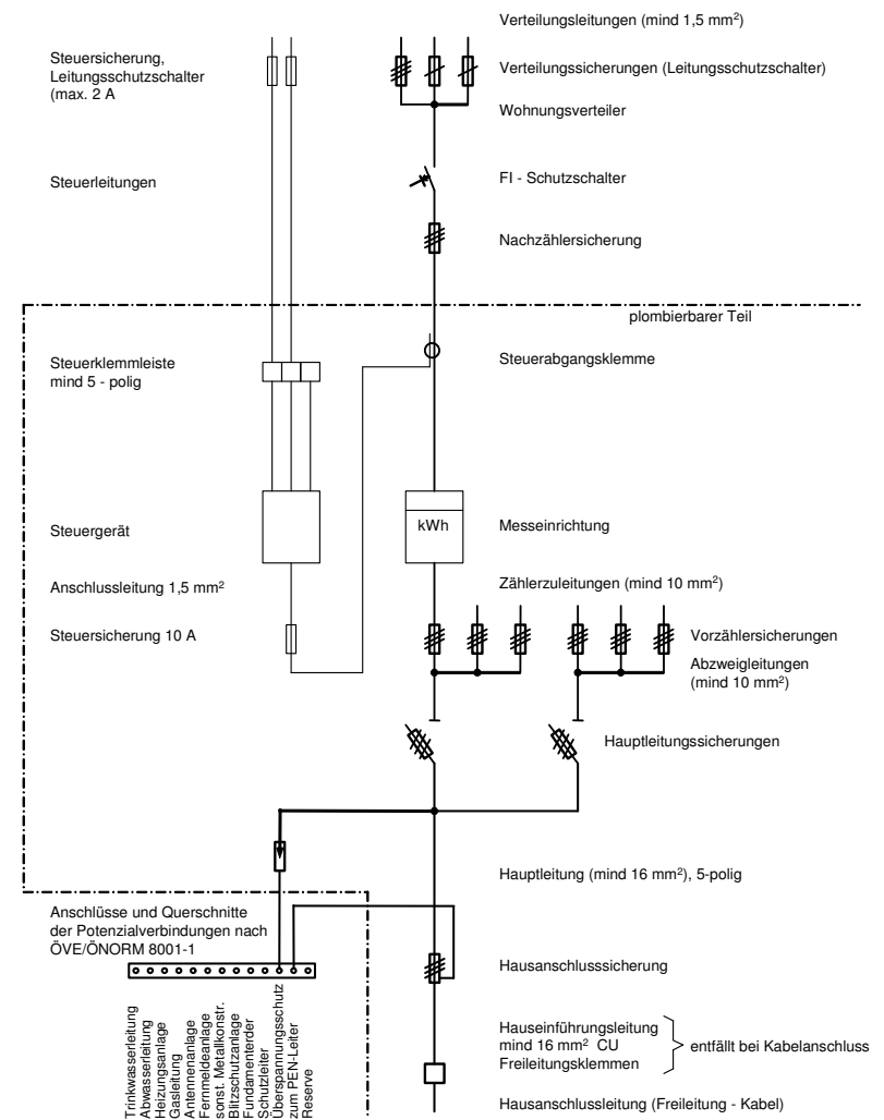
Abb. 1: Begriffsbestimmungen bei der Hausinstallation
